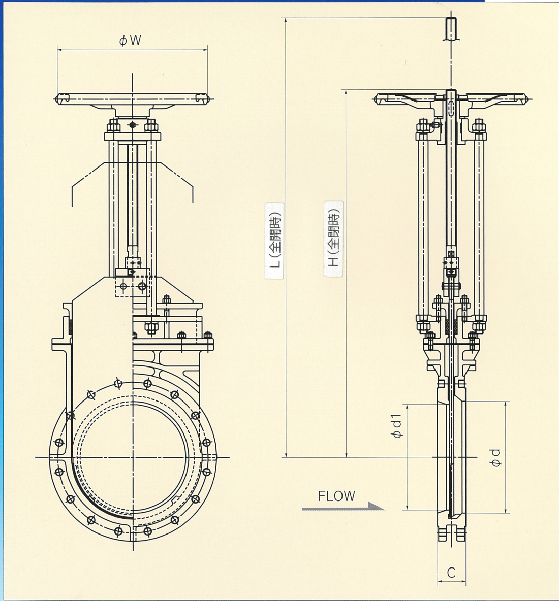
寸法表
