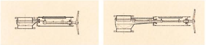
DS-02型 弁板シール型（手動式）
