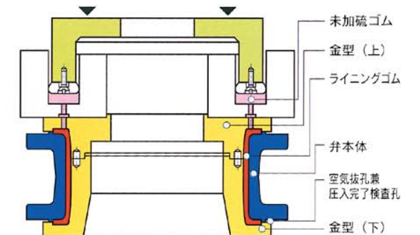
■金型によるゴムの圧入、加硫接着の説明図
