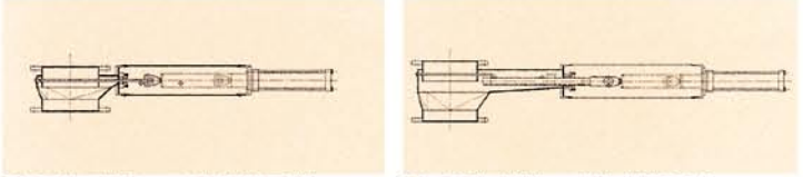
DS-04型 弁板シール型（空気圧式）
